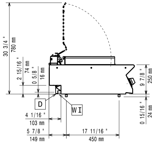
Zij aanzicht
